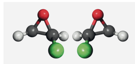
Abb. 2: Struktur von (S)-2-Chloroxiran (links) und (R)-2-Chloroxiran (rechts).
