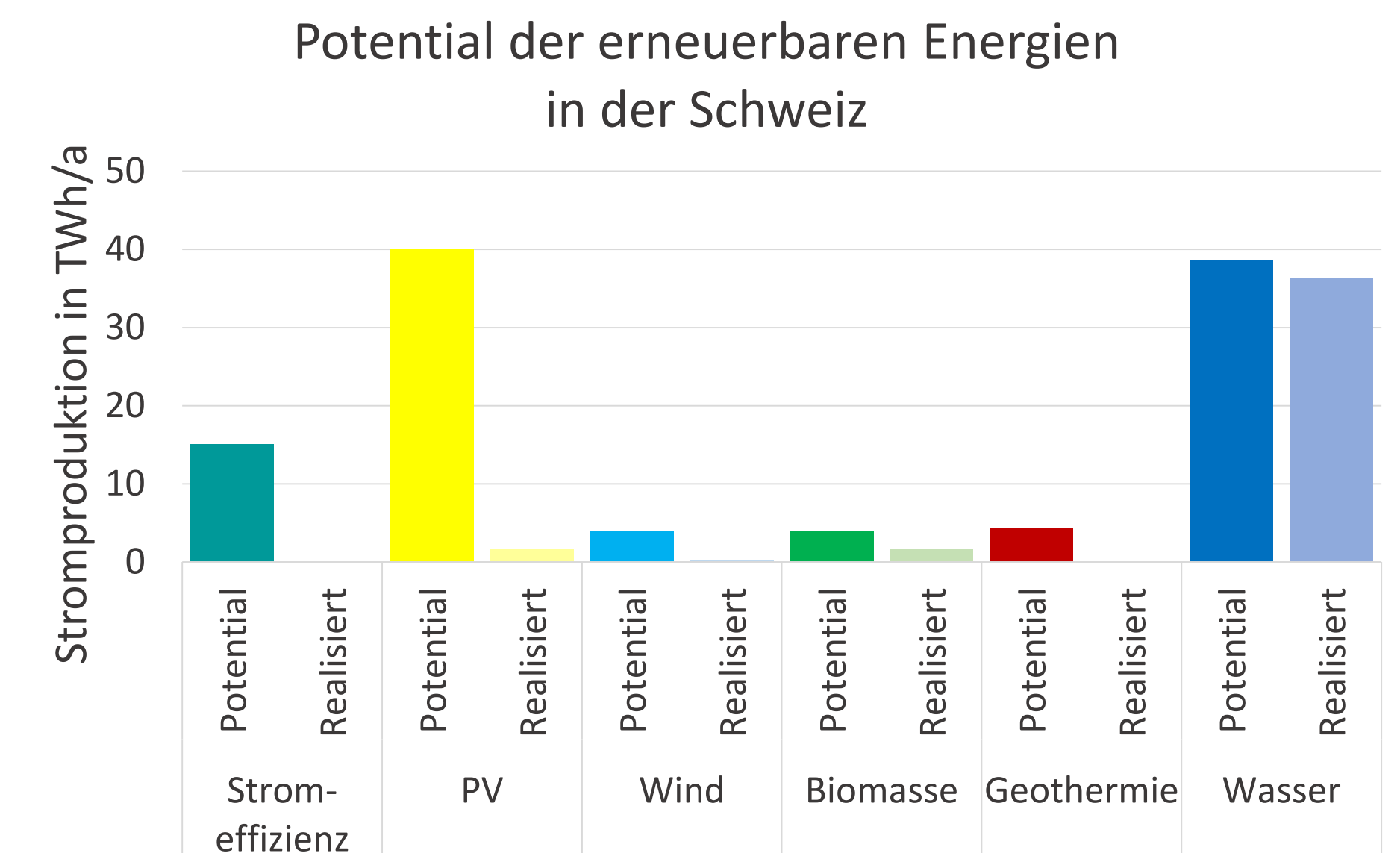
Abb. 4: Potentiale der erneuerbaren Energien und der Stromeffizienz-Massnahmen in der Schweiz bereits realisierte Anteile
